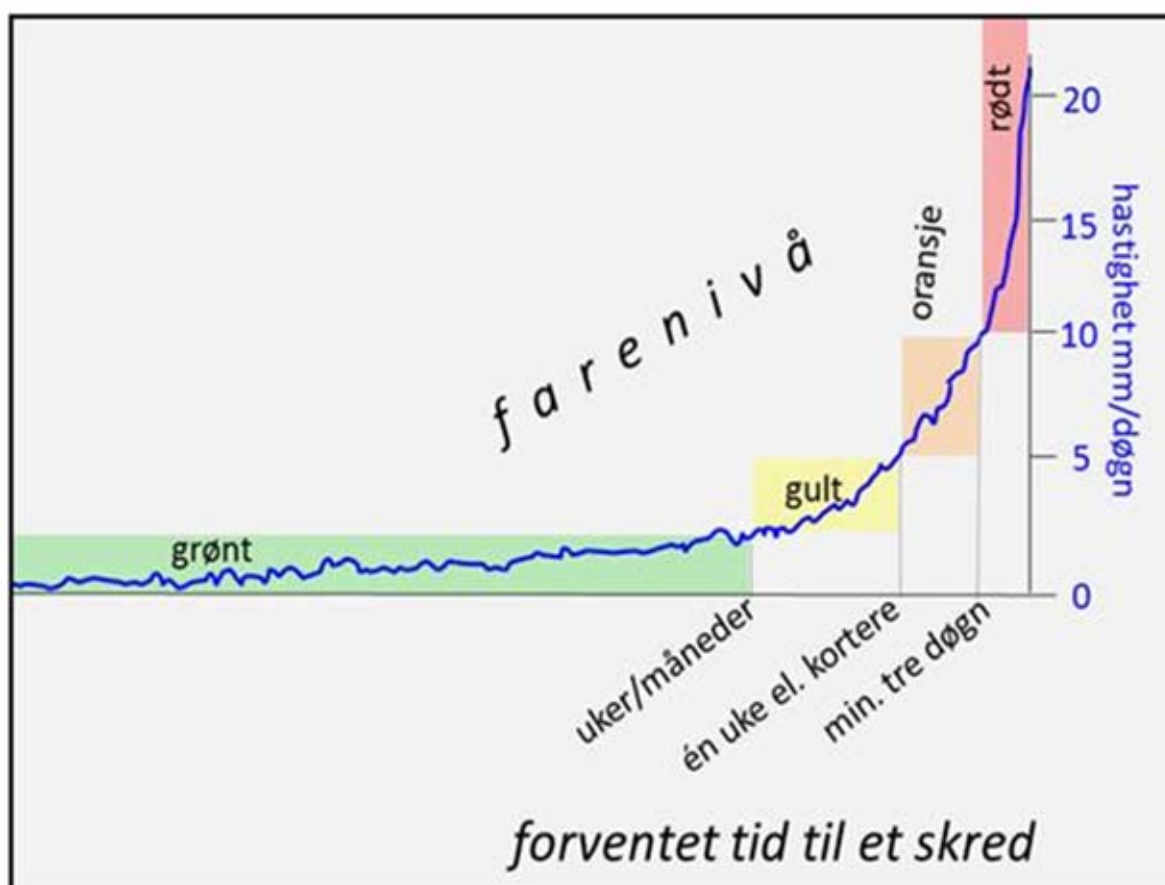
Figur 3.1. Diagram som viser utvikling av et fjellskred gjennom de definerte farenivåene. Fremstillingen er skjematisk. Hvert fjellskred kan ha sin egen utviklingskurve.
